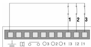
1, 2, 3 - drátové snímače
